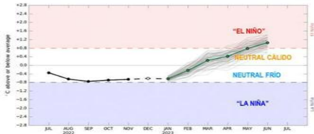
REANÁLISIS Y PRONÓSTICO DE LA EVOLUCIÓN DE LAS ANOMALÍAS DE TEMPERATURA EN LA ZONA "EL NIÑO 3.4", EMITIDA POR EL BOM (AU) EL 31 DE DICIEMBRE DE 2022.
